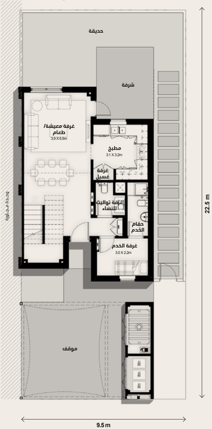
مخطط الطابق الأرضي
