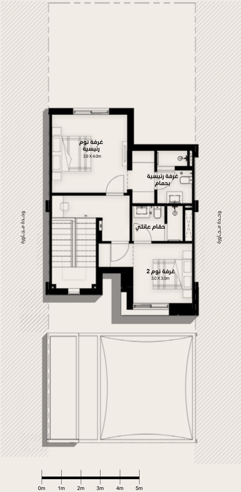
مخطط الطابق الأول
